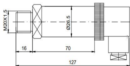
WH 卫生型压力变送器螺纹安装尺寸
