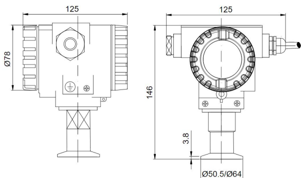
WP 卫生型压力变送器卡箍式快接法兰尺寸
