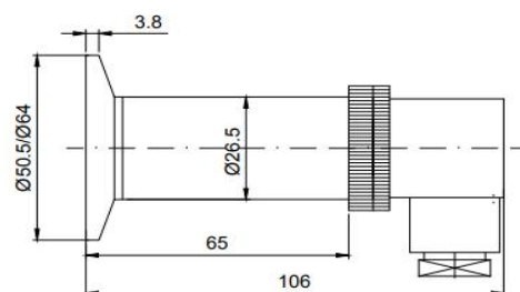
WH 卫生型压力变送器卡箍式安装外形
