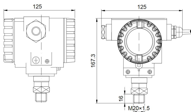
WP 卫生型压力变送器螺纹安装尺寸
