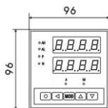
外形尺寸
