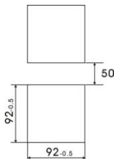
开孔尺寸
